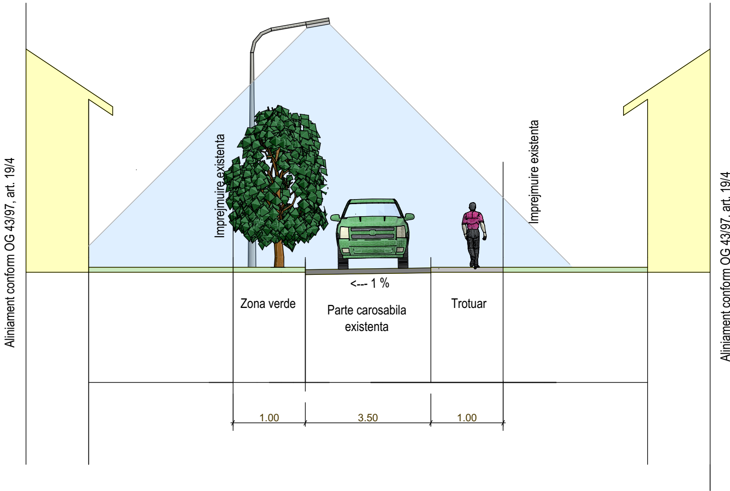
PROFIL TRANSVERSAL TIP IV-IV SCARA 1:100
