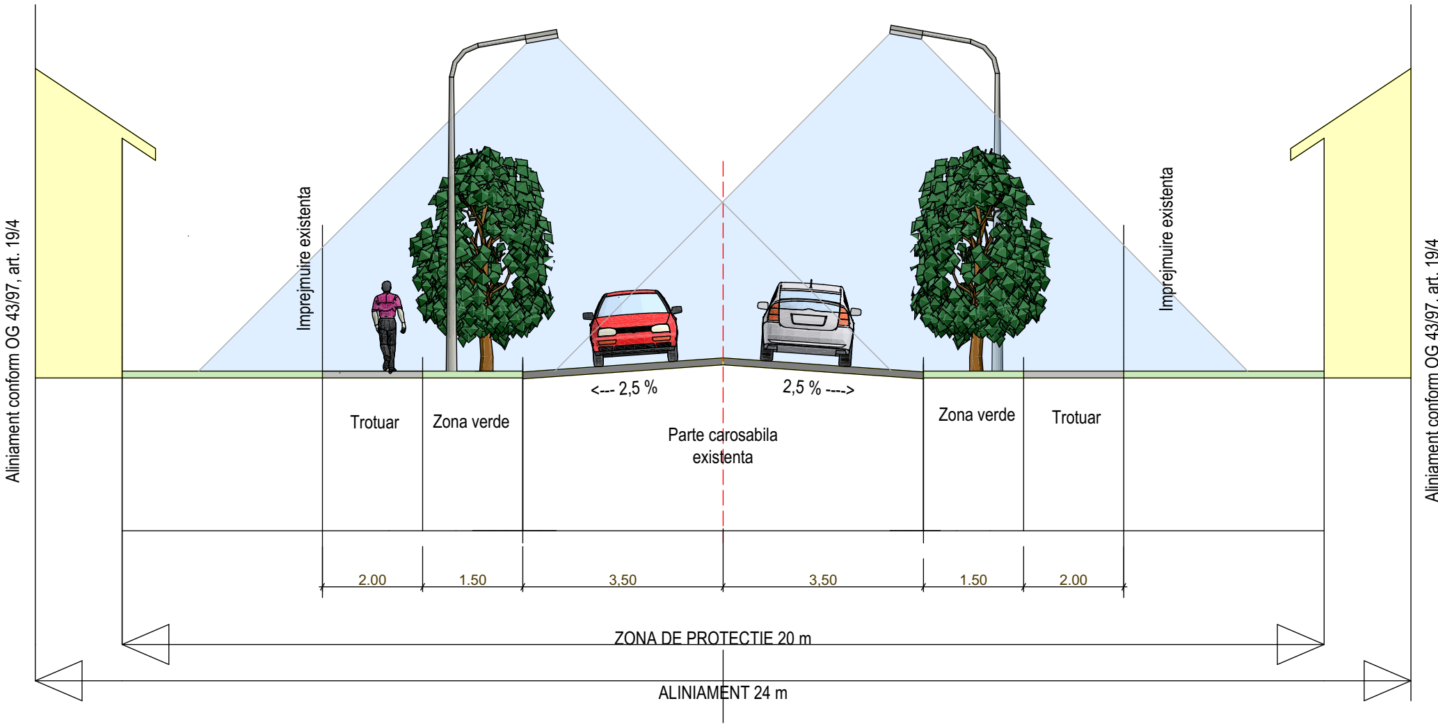
PROFIL TRANSVERSAL TIP I-I PRIN DJ 401A - INTRAVILAN - SCARA 1:100
