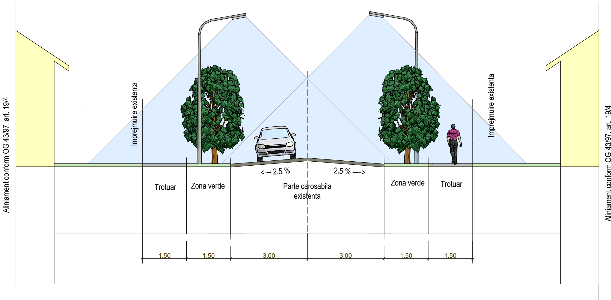
PROFIL TRANSVERSAL TIP III-III SCARA 1:100
